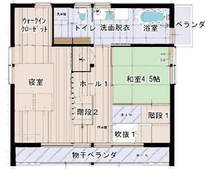
2階平面図
